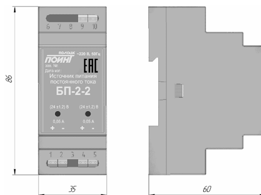
Рисунок 8.1 – Источник питания постоянного тока БП-2 двухканальный
