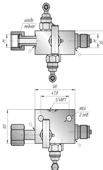
Клапан КЗИК-И-23.X3-15-400-M-S
