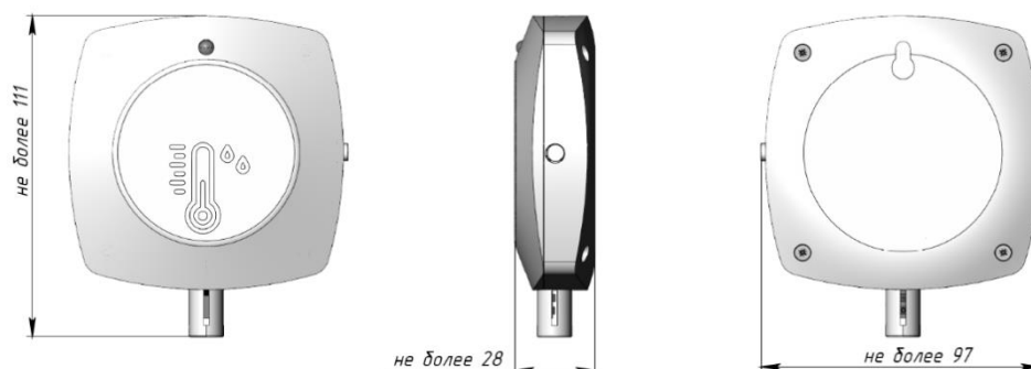
Рисунок 7.3-Прибор измерительный ПИ-002/11М,ПИ-002/11М.Д
