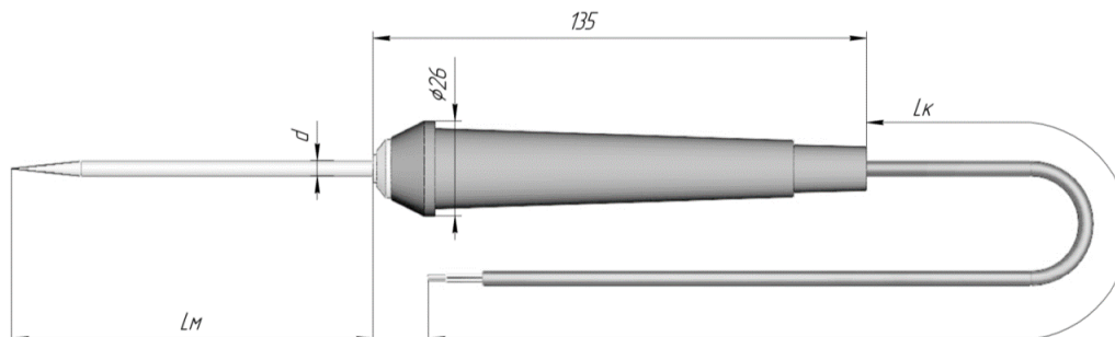
Рисунок 7.4 – Щуп для измерения температуры продуктов питания*
