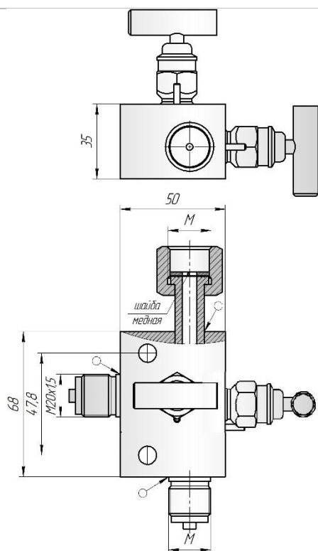
Клапан КЗИК-33.X2-15-400-M-S
