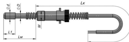
Термопара с кабелем «Б», с кабельной угловой монтажной частью «Ky»
