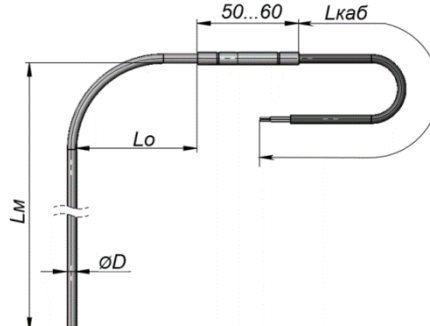
Термопара с кабелем «Б», с кабельной угловой монтажной частью «Ky»
