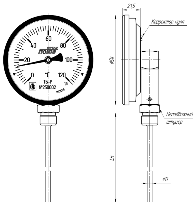
Рисунок 4.2 – Радиальное исполнение
