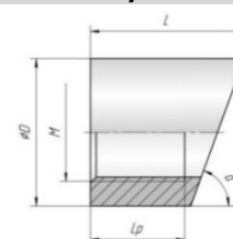
Бобышка 2/D - L - M/a - S
