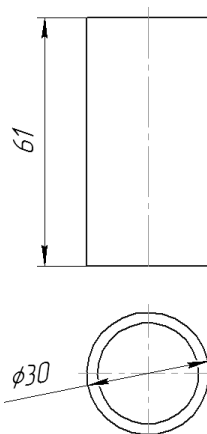
Масса не более 0,1 кг. Рисунок 10.1 – Респондер
