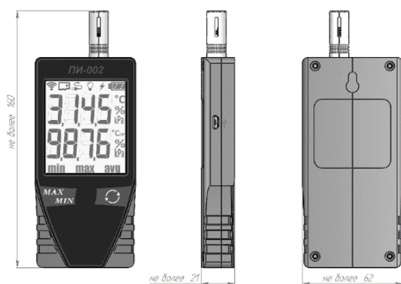
Рисунок 7.1-Прибор измерительный ПИ-002/1М, ПИ-002/1М.Д, ПИ-002/2М, ПИ- 002/2М.Д
