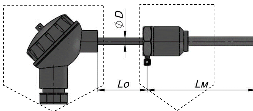
Исполнение клеммной головы
