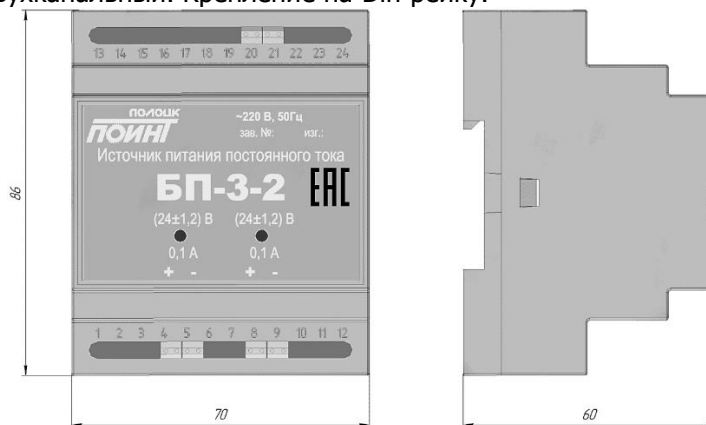
Рисунок 8.2 – Источник питания постоянного тока БП-3 двухканальный
