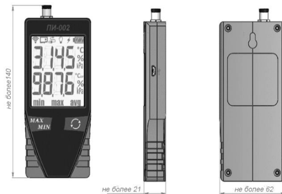
Рисунок 7.2 - Прибор измерительный ПИ-002/3М, ПИ-002/4М
