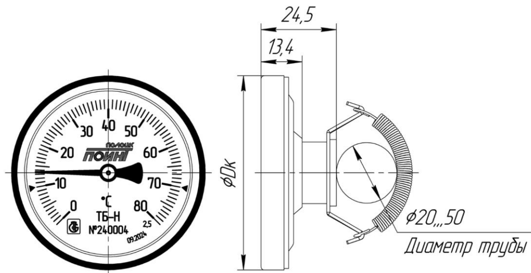
Рисунок 3.4 – Накладное исполнение
