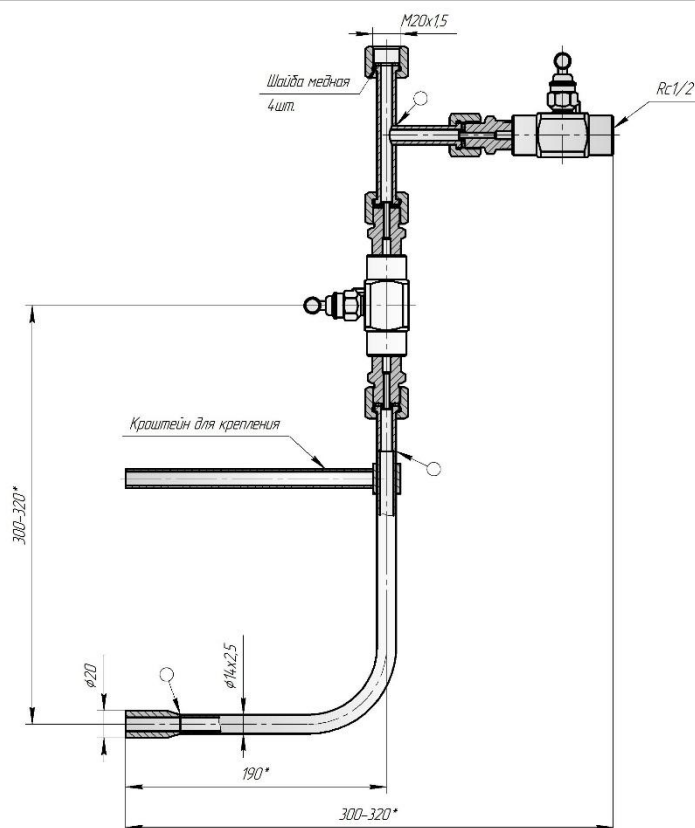
Манометрическая сборка ОУД - 16 - Т - Н - S (X)
