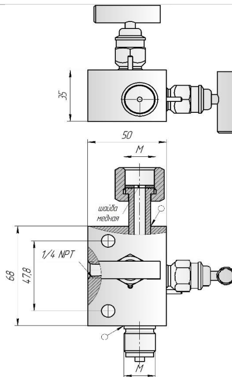
Клапан КЗИК-23.X2-15-400-M-S
