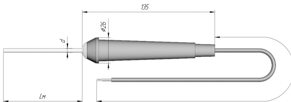
Рисунок 7.5 – Щуп для измерения температуры сыпучих материалов*
