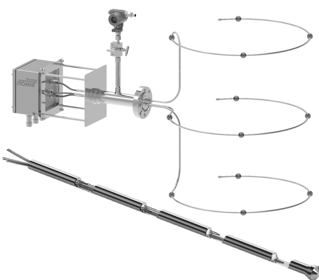
Рисунок 3.4 - Термопара для измерения температуры в слоях катализатора гидрокрекинга (в одной защитной оболочке находится до 16 точек измерения, материал оболочки выполнен из материалов, стойких к измеряемой среде: AISI 347; AISI 316L)
