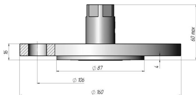
Φ-ΦP-DN50/PN16/E-316L/904L-PFA-BT
