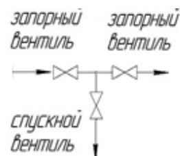
Клапан КЗИК-И-23.X3-15-400-M-S
