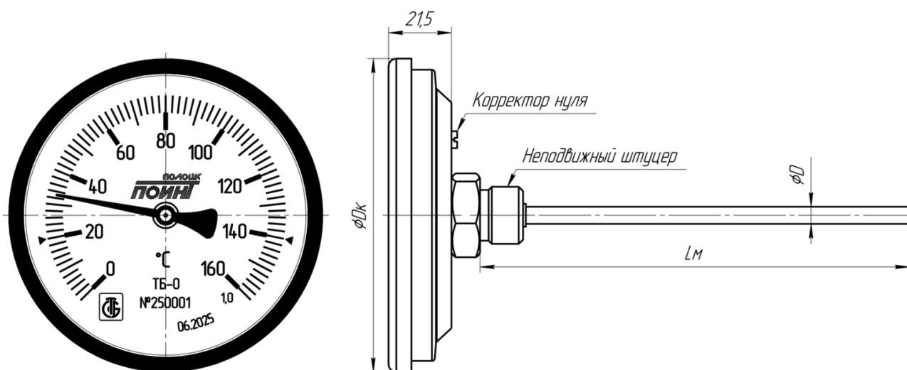
Рисунок 4.1 – Осевое исполнение
